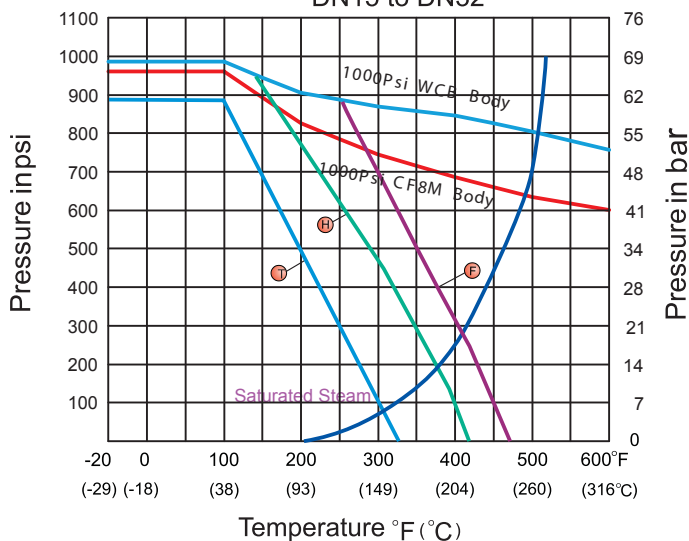
Full Bore : NPS ½ ~ NPS 1 ¼ DN15 to DN32
